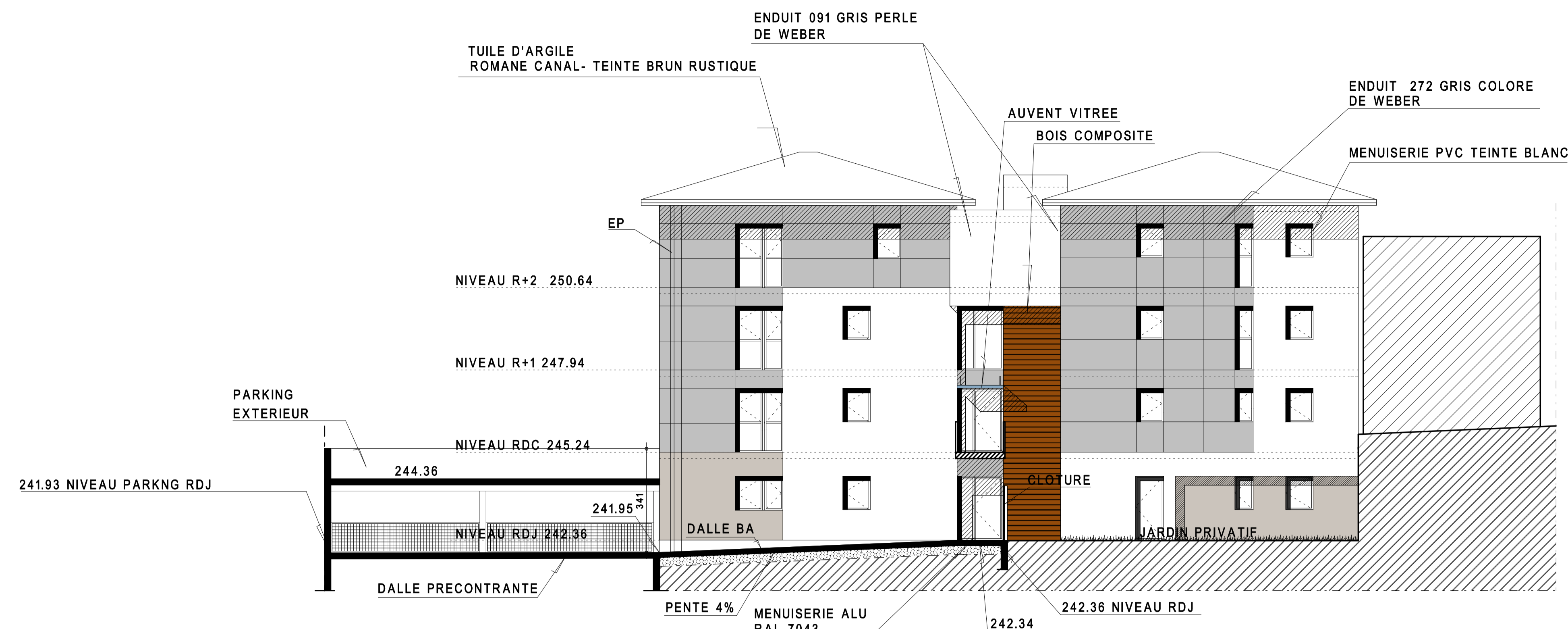
FACADE SUR ENTREE RDJ ECHELLE 1/100
